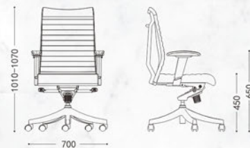
Dimensions 外形尺寸图
