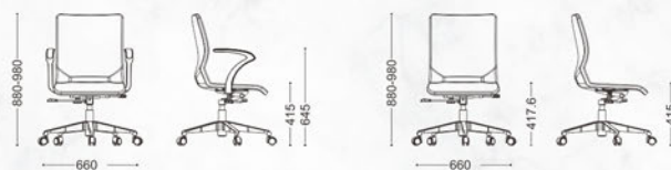
Dimensions 外形尺寸图
