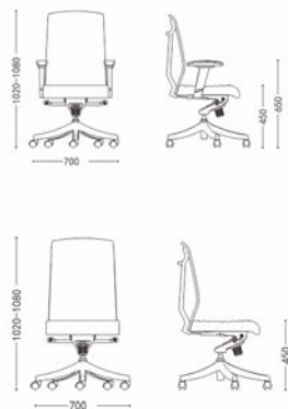
Dimensions 外形尺寸图
